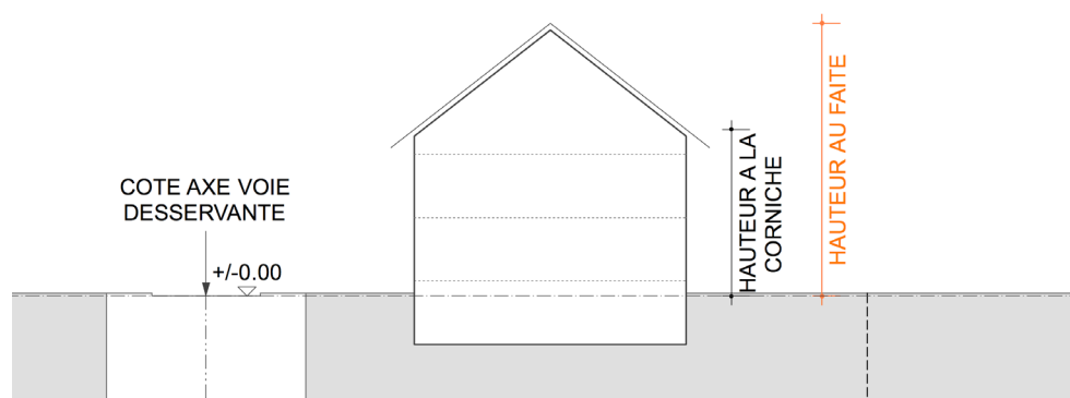
Figure 15.23: Hauteur au faîte
