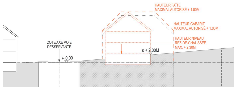
Figure 14.2.2.1.1 : Topographie accidentée ascendante
