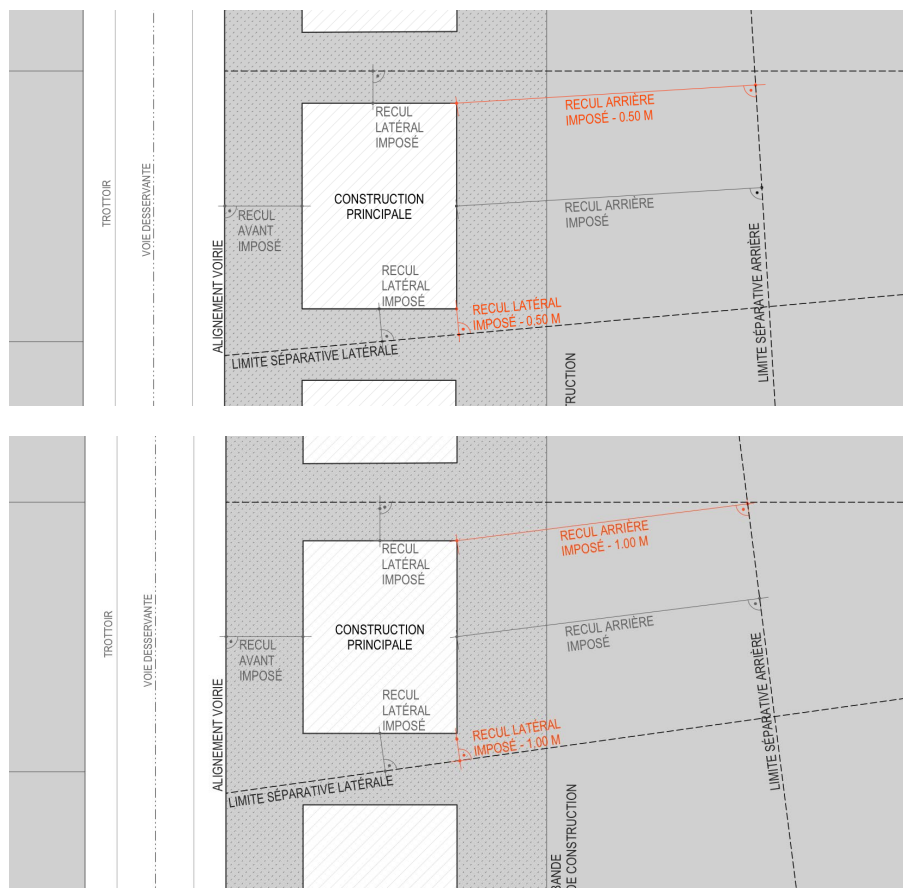
Figures 14.5.1 : Reculs par rapport à des limites parcellaires obliques
