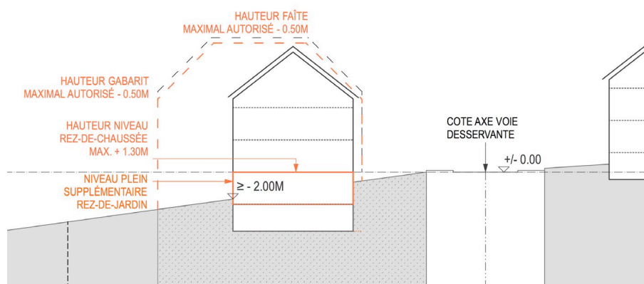
Figure 14.2.2.1.2 : Topographie accidentée descendante
