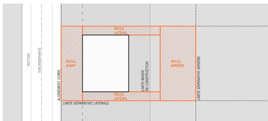
Figure 15.45 : Reculs des constructions
