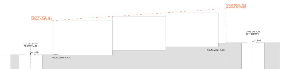
Figure 14.2.2.2.3 : Deux voies desservantes de cotes différentes
