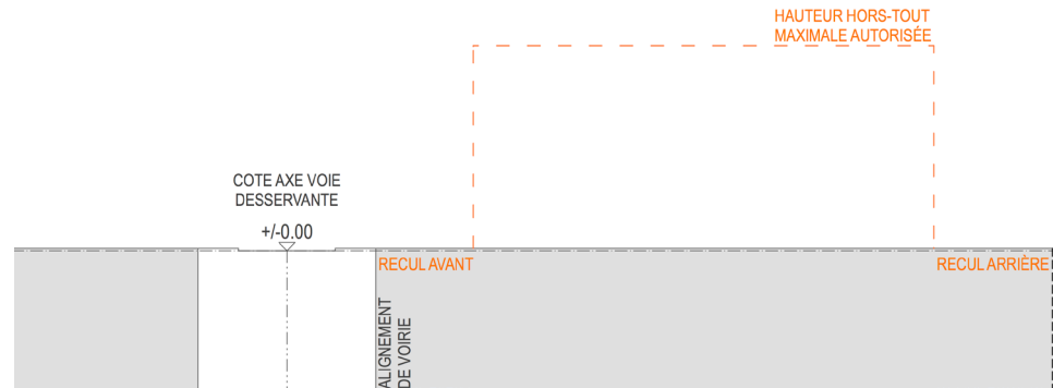
Figure 15.20.3: Vue en coupe du gabarit de construction maximal autorisé des quartiers existants situés dans les zones MIX-r, GARE, REC BEP, ECO-c1 et 2, COM et SPEC-1
